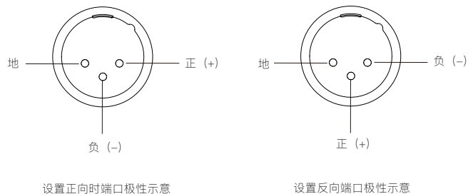
设置正向时端口极性示意
