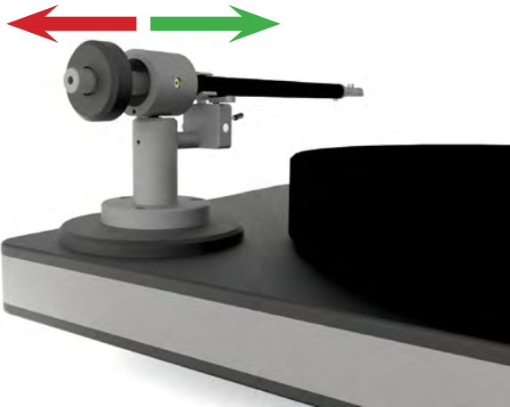
Abb. 13: Einstellen des Auflagegewichts
