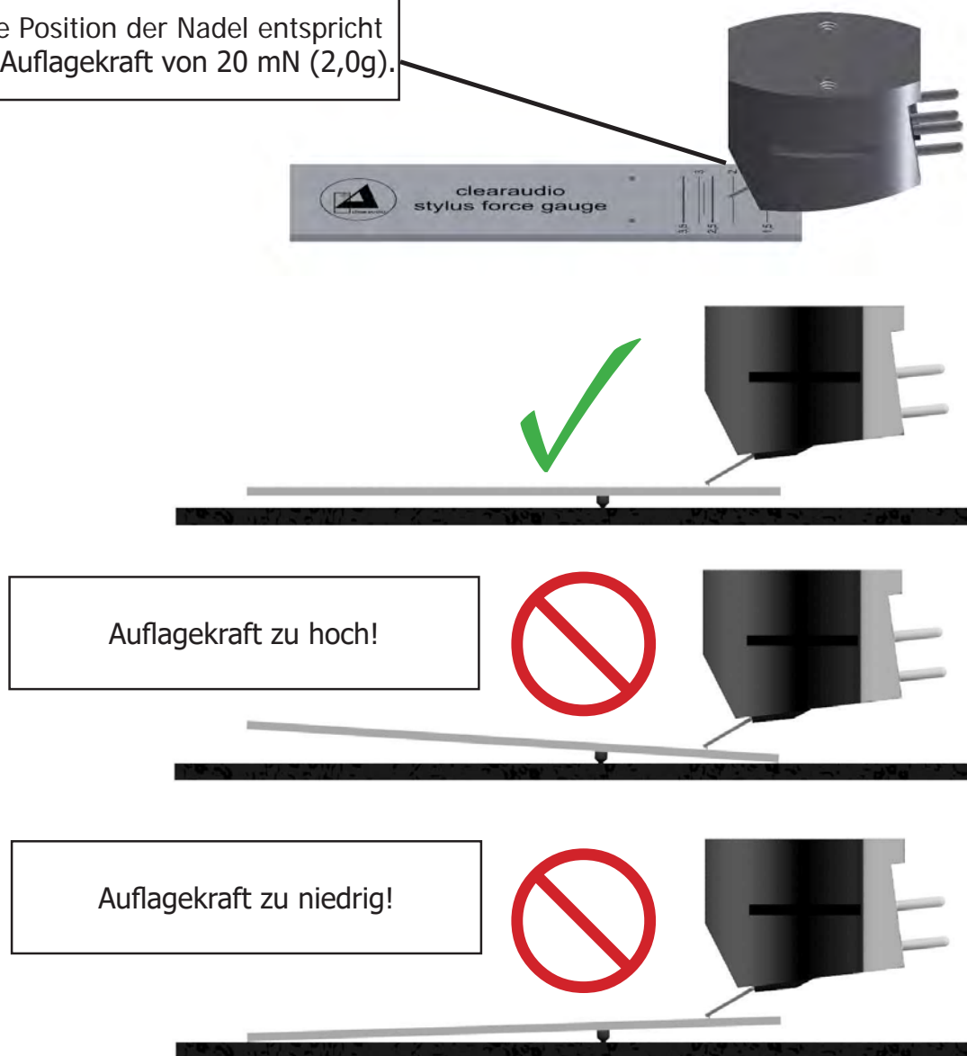
Abb. 11: Benutzung der Kippelwaage
