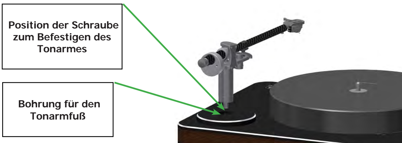
Abb. 10: Rückansicht Clarify Tonarm
