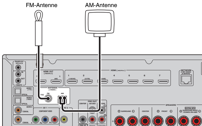
Gerät (Rückseite)
